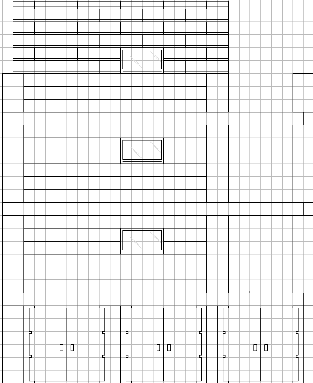
AANZICHT - RECHTERZIJDE
